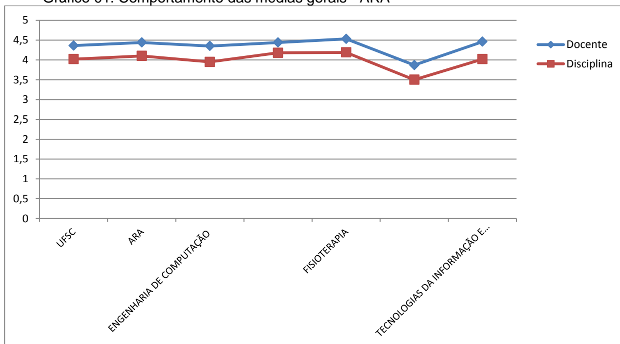
Gráfico 01: Comportamento das médias gerais - ARA
