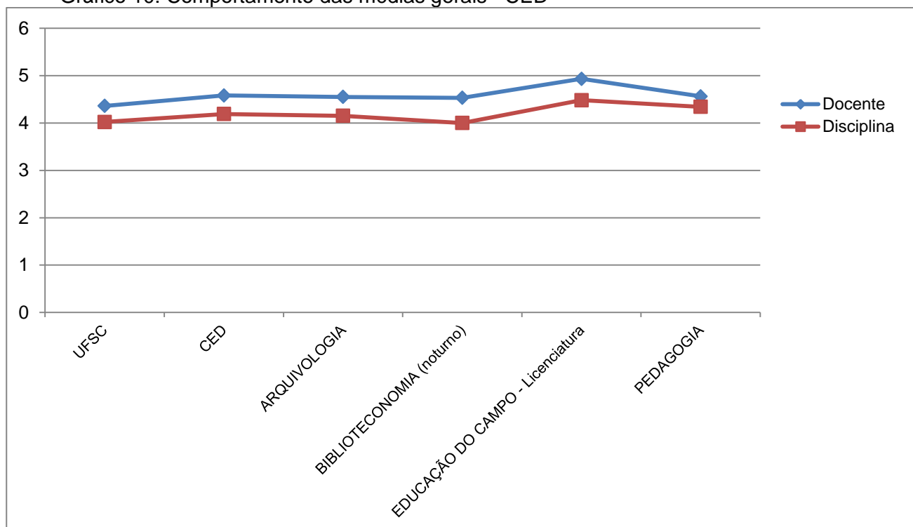
Gráfico 10: Comportamento das médias gerais - CED
