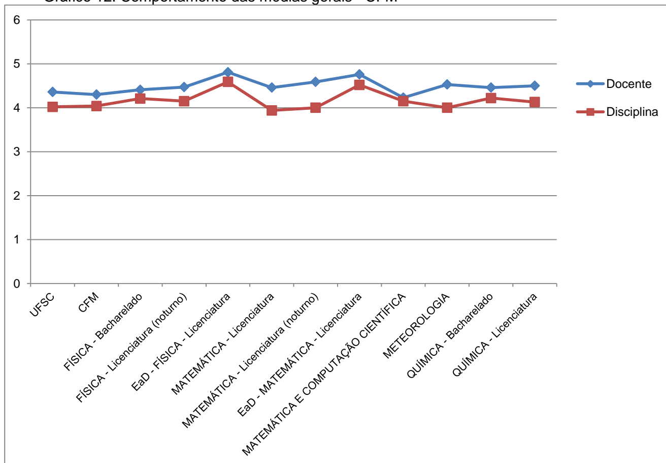
Gráfico 12: Comportamento das médias gerais - CFM
