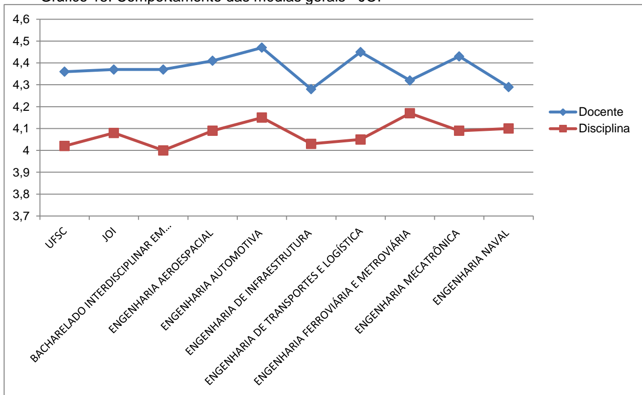
Gráfico 15: Comportamento das médias gerais - JOI
