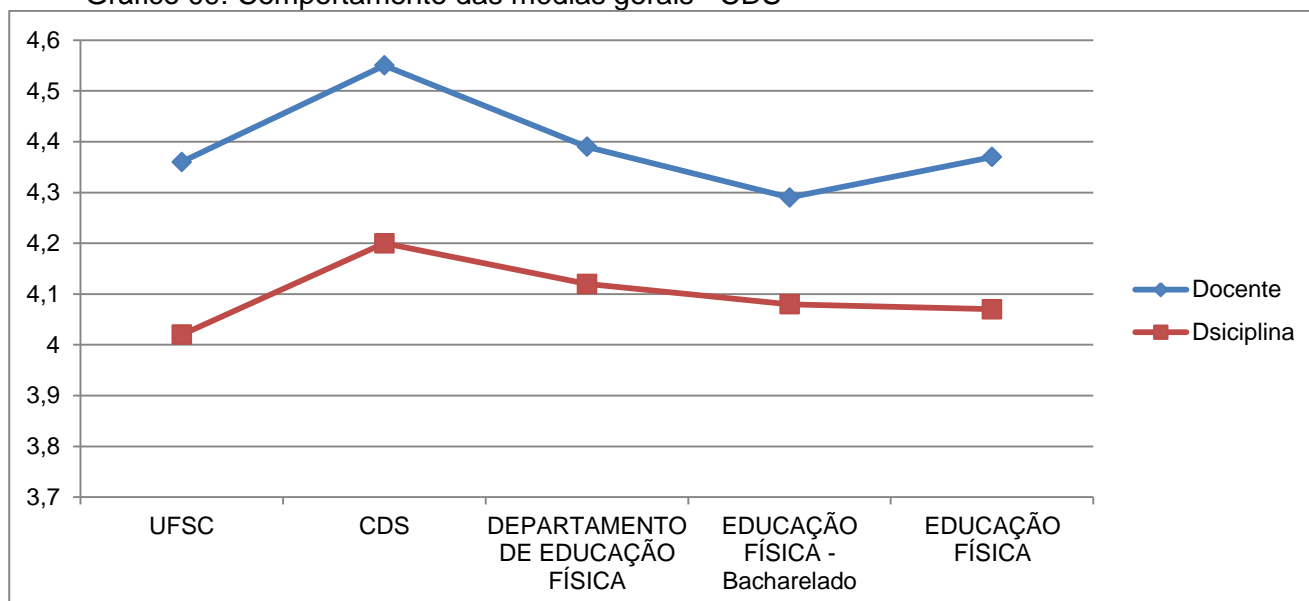
Gráfico 09: Comportamento das médias gerais - CDS
