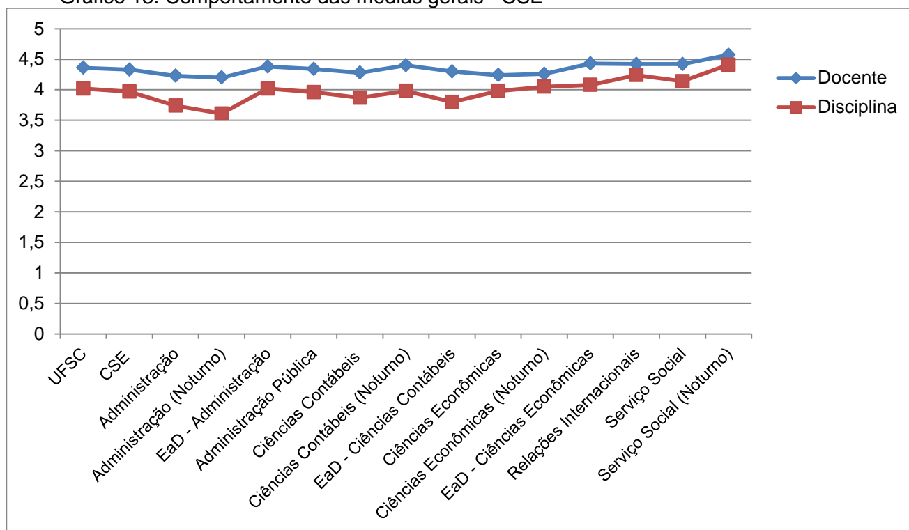
Gráfico 13: Comportamento das médias gerais - CSE
