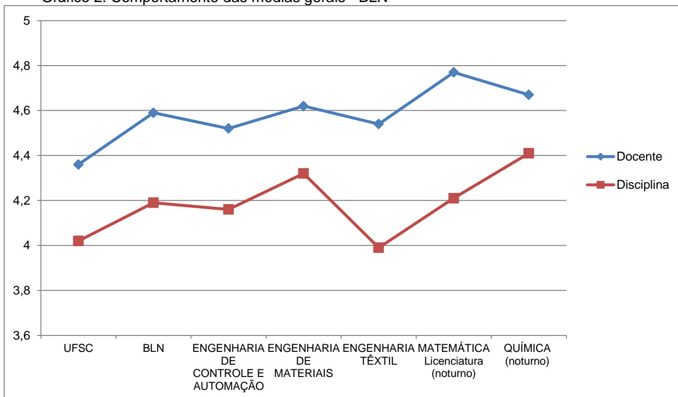
Gráfico 2: Comportamento das médias gerais - BLN
