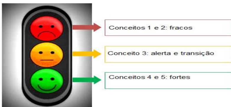
Figura 01: Pressupostos da CPA
