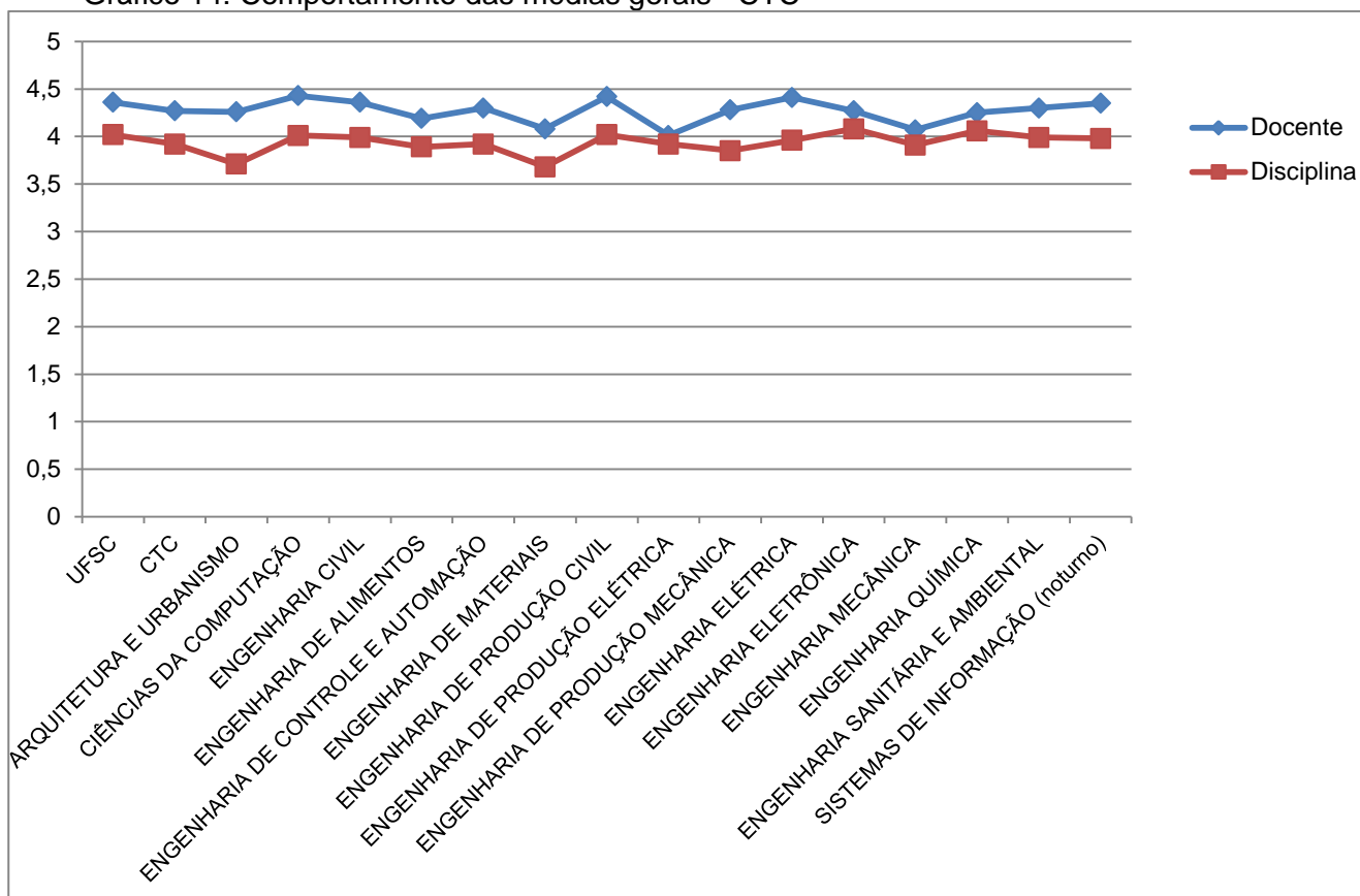
Gráfico 14: Comportamento das médias gerais - CTC
