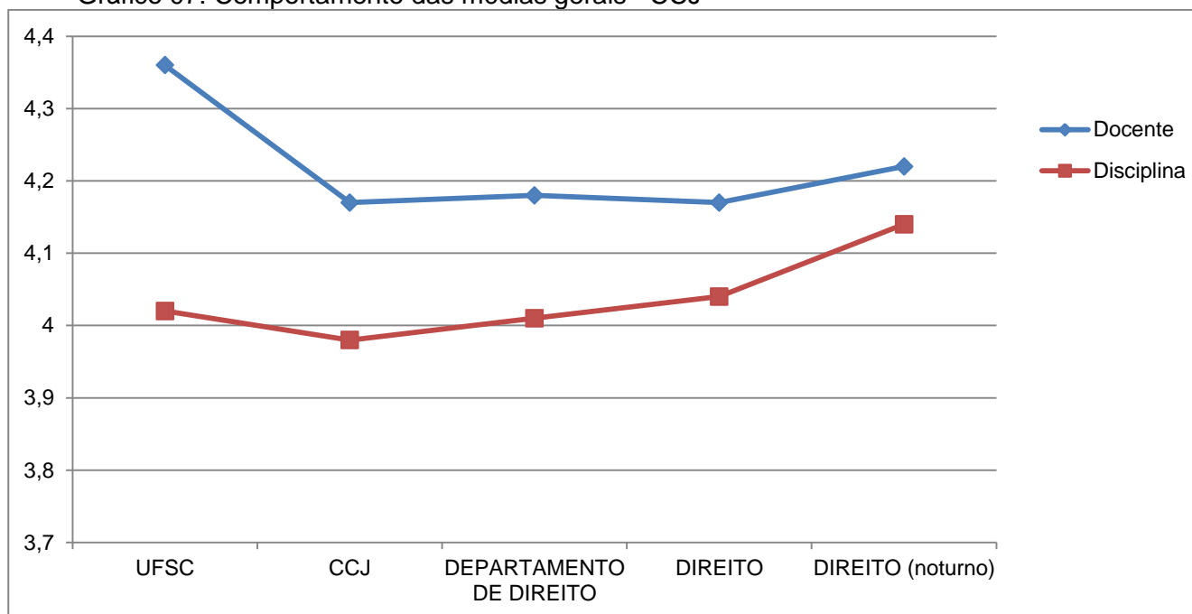
Gráfico 07: Comportamento das médias gerais - CCJ
