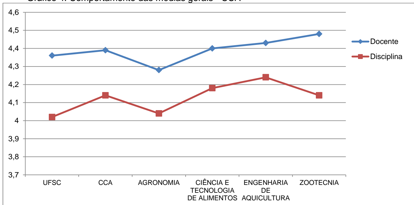
Gráfico 4: Comportamento das médias gerais - CCA
