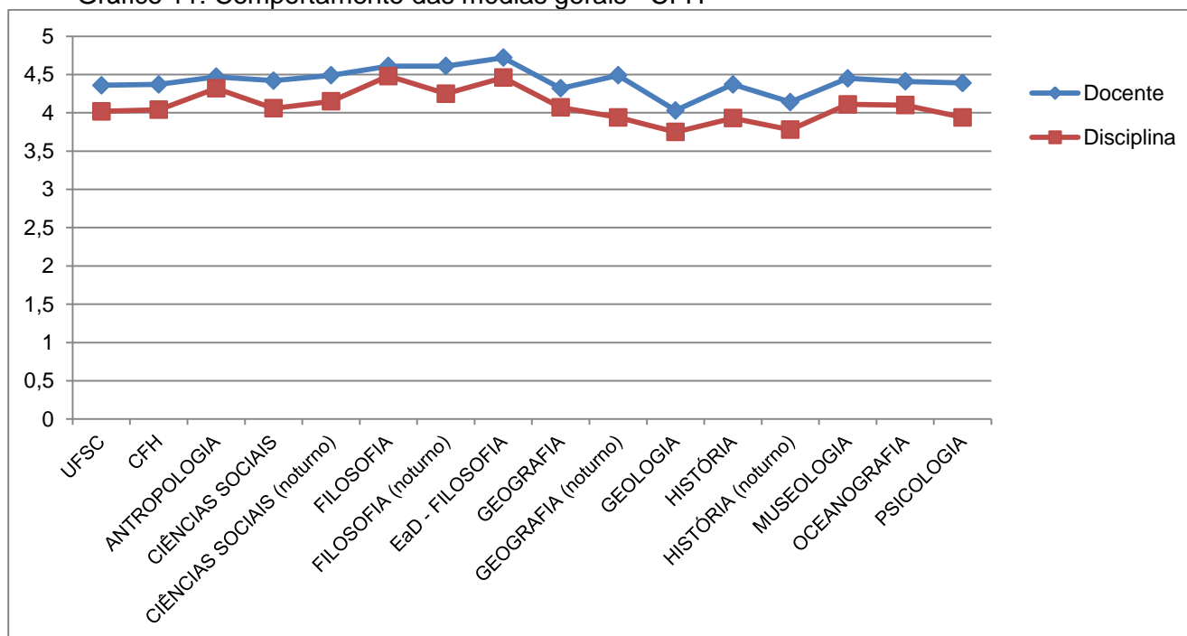
Gráfico 11: Comportamento das médias gerais - CFH
