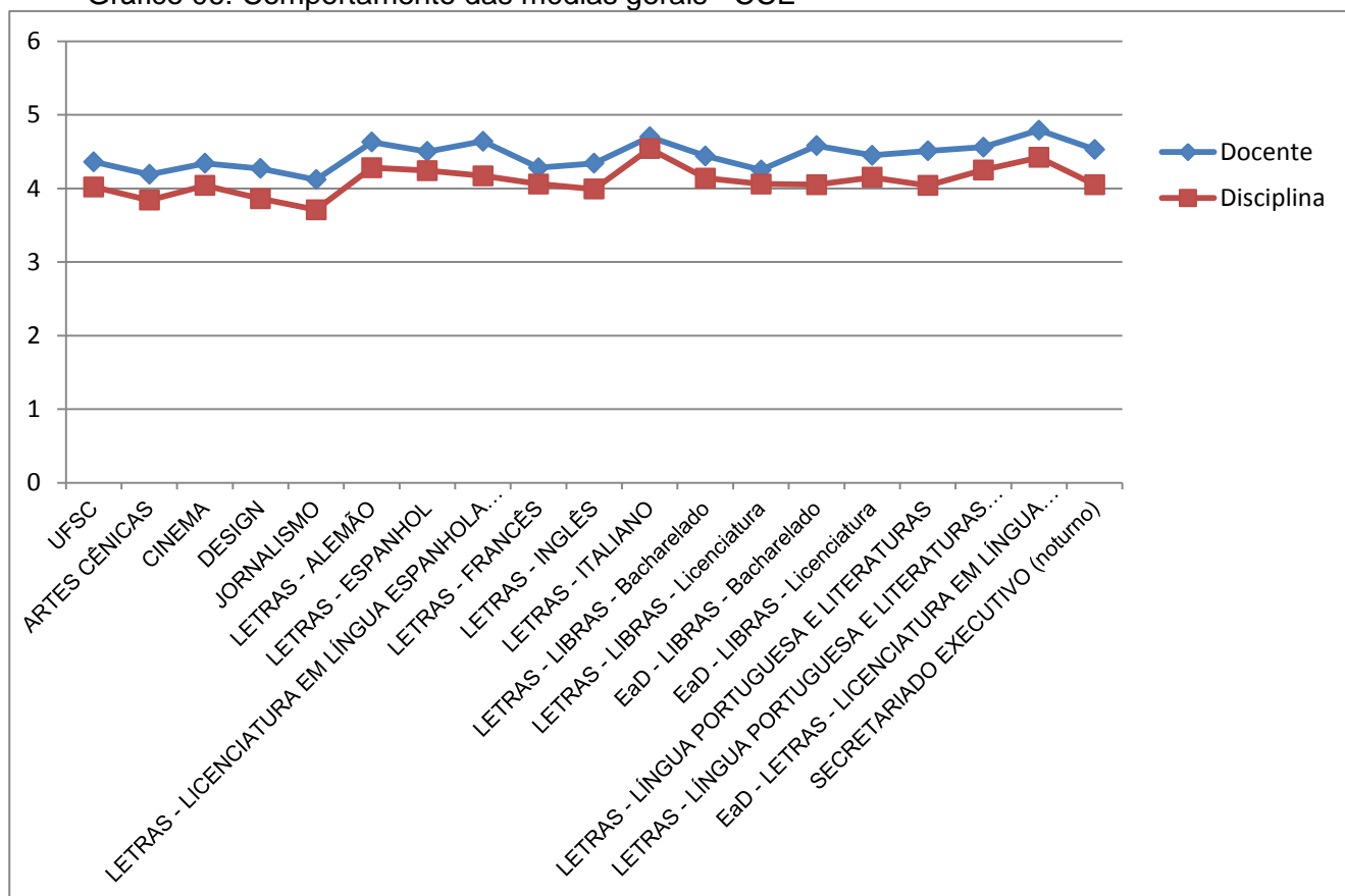
Gráfico 06: Comportamento das médias gerais - CCE
