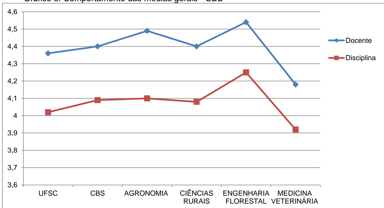
Gráfico 3: Comportamento das médias gerais - CBS
