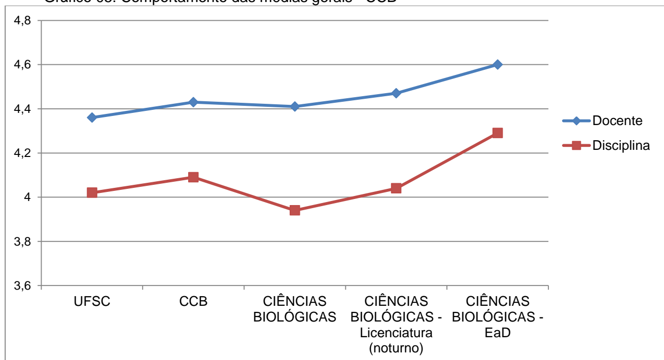
Gráfico 05: Comportamento das médias gerais - CCB
