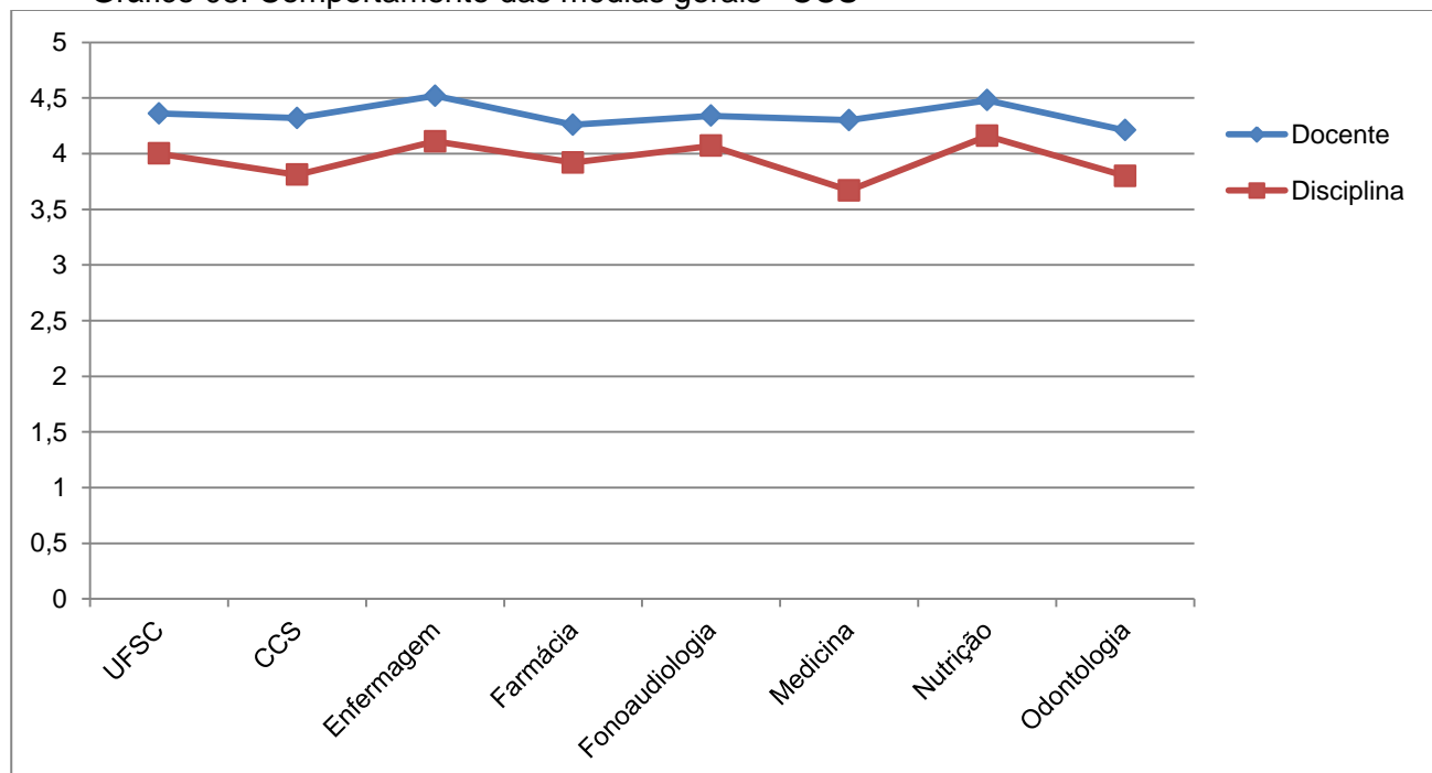
Gráfico 08: Comportamento das médias gerais - CCS
